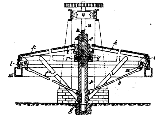
20879 Rheinisch-Nassauische Bergwerks and Hütten-Actien-Gesellschaft. Ore-dresser. (Demuth.)
